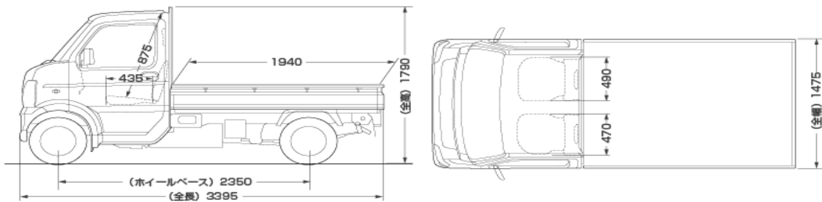
寸法図 KC
